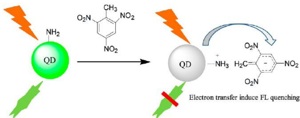
شکل ۵- مکانیزم خاموش شوندگی QDs بر اساس انتقال انرژی رزونانسی فلئورسنسی (FRET) (۲۲)
