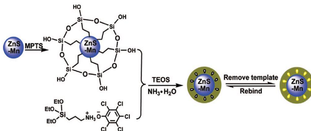
شکل ۷- نمایش شماتیک برای ساخت نقاط کوانتومی ZnS پوشیده شده با Mn پوشیده شده با پلیمرهای قالب مولکولی (MIP-capped Mn-ZnS QDs) (۲۴).
