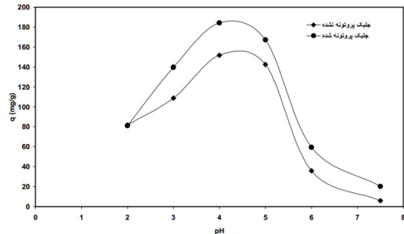
شکل ۵- تاثیر pH بر میزان جذب تعادلی اورانیوم توسط جلبک قهوه‌ای سیستوسریا ( غلظت اولیه ppm ۳۵۰، غلظت جاذب g/L ۲، دما °C ۳۰، سرعت هم‌زدن rpm ۱۵۰) (۱۳).
