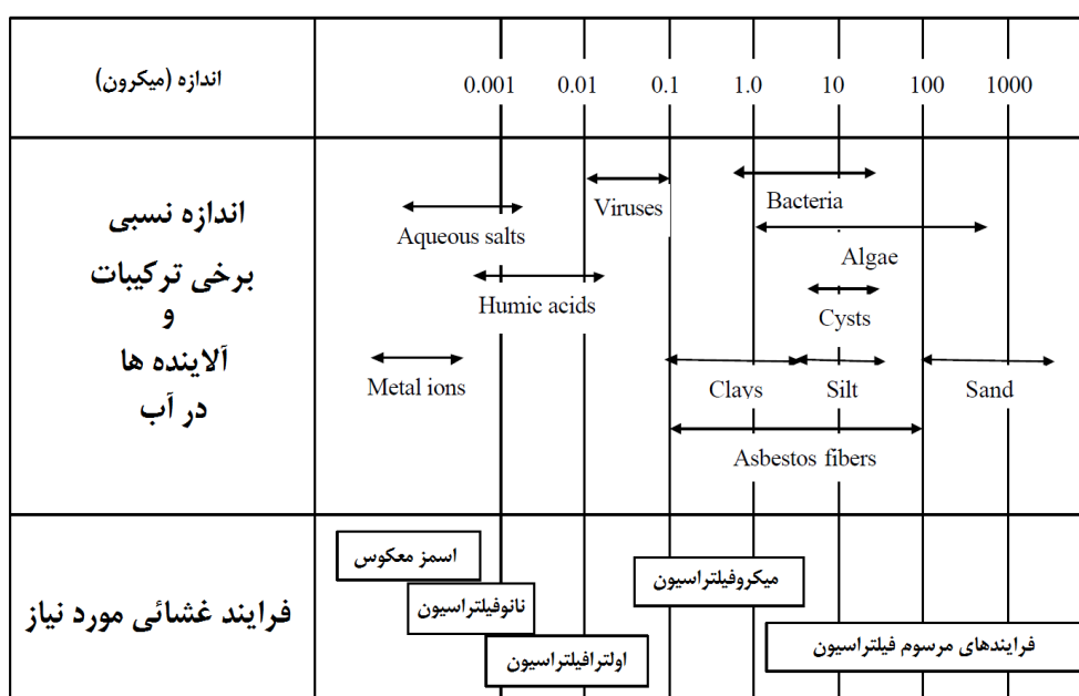
شکل ۳- بررسی محدوده کاربرد فرایندهای غشائی برای حذف برخی ترکیبات مرسوم موجود در آب
