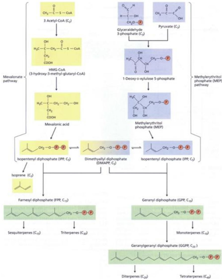
شکل ۲- نمایش فهرست‌وار زیست‌ساختی‌ترین‌ها. واحدهای ۵ کربنی پایه‌ترین‌ها از دو مسیر ساخته می‌شوند. ترکیبات حد واسطه فسفریله شده IPP و DMAPP برای ساختن‌ترین‌های ۱۰ و ۱۵ کربنه و‌ترین‌های بزرگ‌تر باهم ترکیب می‌شوند.
