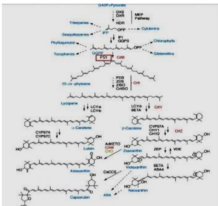
شکل ۱- مسیر عمومی بیوسنتز کاروتنوئیدها در گیاهان. نام ترکیبات به رنگ آبی و نام آنزیم‌ها به رنگ سیاه (آنزیم‌های گیاهی)، قرمز (آنزیم‌های باکتریایی) و سبز (از جلبک سبز و سیانوباکترها) می‌باشد (۵).
