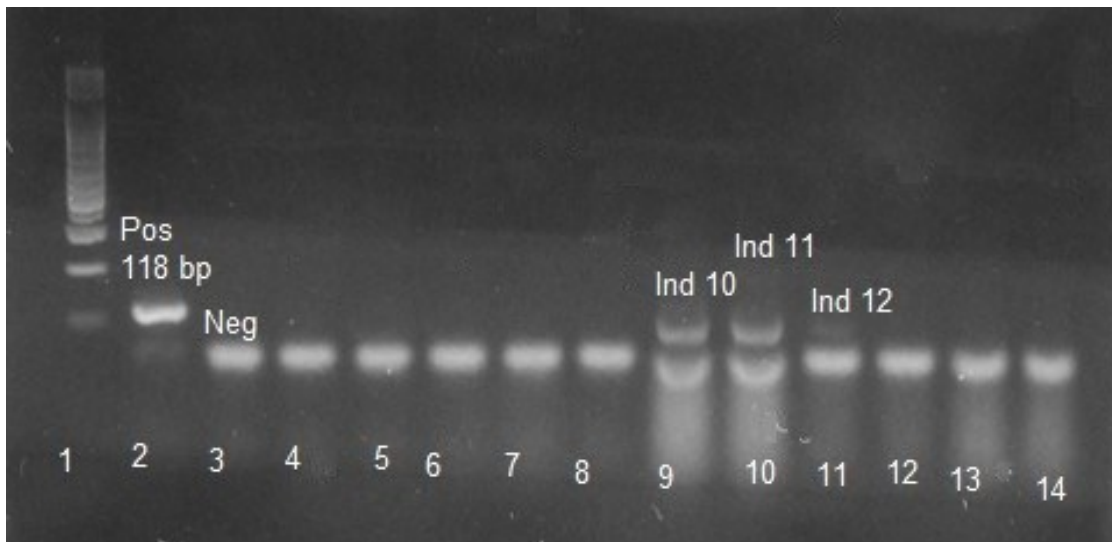
شکل ۳- غربال گری نمونه ها با استفاده از توالی پایانبر NOS (۱۱۸ bp)
