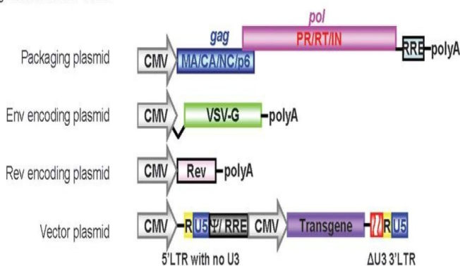
شکل ۵- سیستم بسته‌بندی لنتی ویروسی نسل سوم (۲۵)
