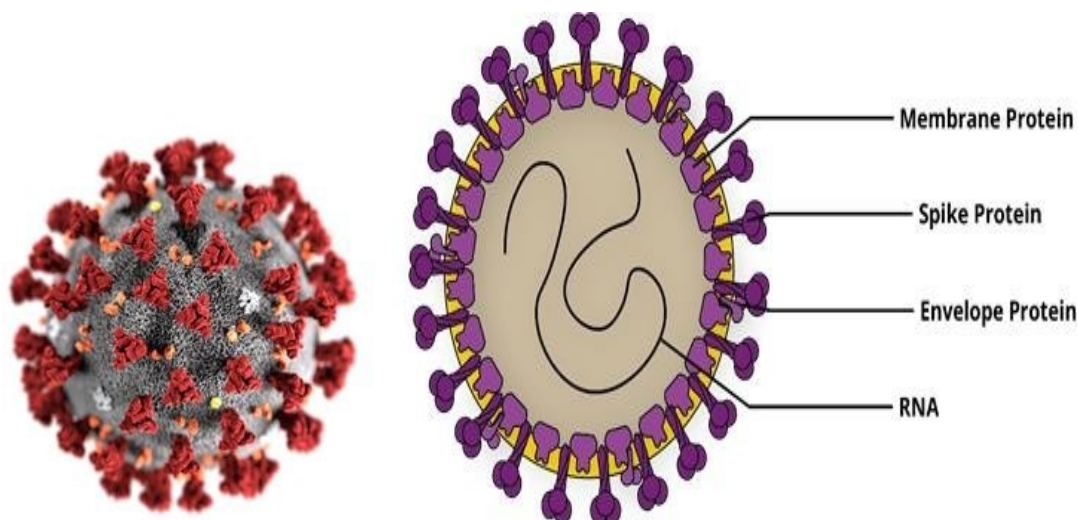
شکل ۱- ساختار و اجزای ویروس کرونا SARS-CoV-2 عامل بیماری COVID-19. ساختار کلی ویروس شامل یک کپسول گلیکوپروتئینی همراه با میخچه‌های از جنس پروتئین (spike) و یک تک‌رشته آر.ان.ا (مثبت) که کدکننده پروتئین‌های حیاتی برای عفونت ویروسی است (۱).
