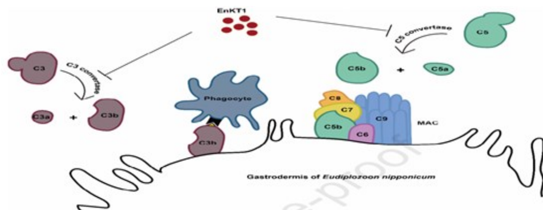
شکل ۲- مهار فعال‌سازی سیستم کمپلمان توسط E. niponicum (Ilgová et al. 2021).
