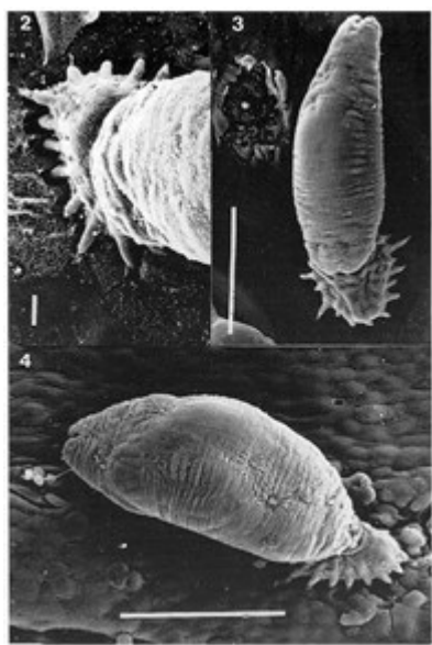
شکل ۱- عکس میکروسکوپ الکترونی از استقرار ژایروداکتیلوس در جاوینی ( Gyrodactylus dergavini ) روی ماهی قزل آلا. نفوذ قلاب‌های انگل در سلول‌های اپیدرم ماهی، تخریب اپی‌تلیوم دم ماهی و ترشح موادی در ناحیه دهان انگل در شکل‌ها مشخص است (Buchmann, 1999).
