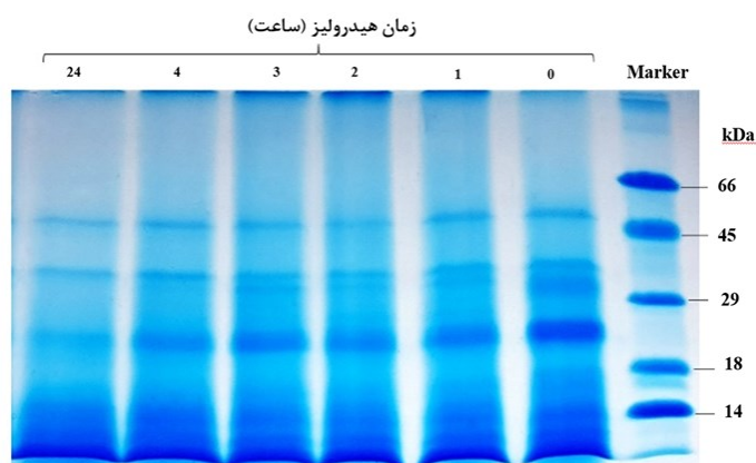
شکل ۱- آزمون الکتروسکوپی به روش OPA (الف) و الکتروفورز ژل پلی آکریلامید (ب) پروتئین کینوا پس از ۱، ۲، ۳، ۴ و ۲۴ ساعت هیدرولیز با آنزیم آلكالاز.
