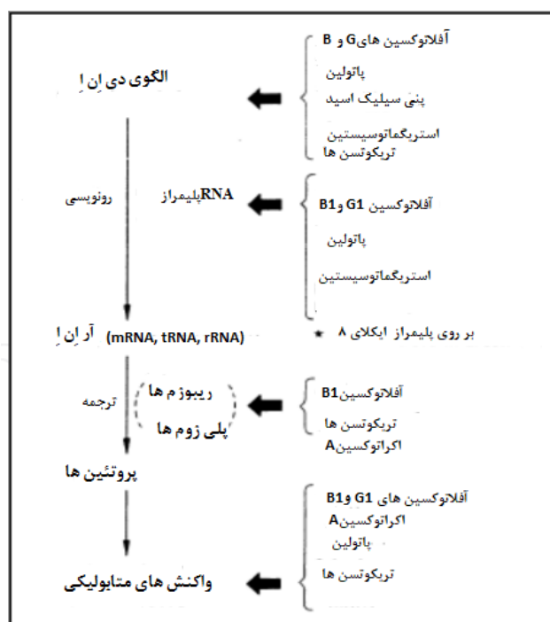
شکل ۱- مکان های مهم تأثیرپذیر توسط برخی از مایکوتوکسین ها (Kiessling. 1986).
