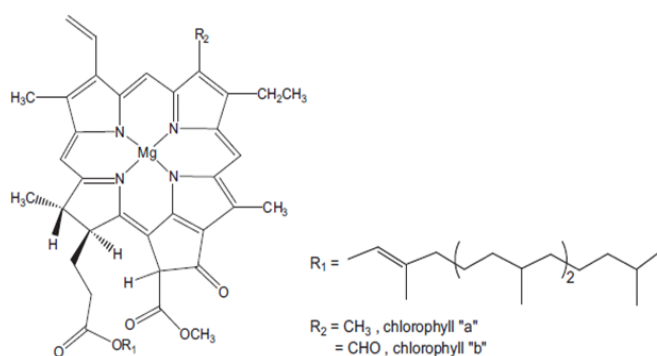
شکل ۲- ساختارهای شیمیایی کلر و فیل (a و b (Pai et al. 2015).
