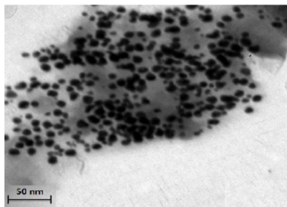
شکل ۴- تصویر میکروسکوپ الکترونی عبوری نانوذرات طلا سنتز شده، با استفاده از عصاره آبی گیاه نعناع فلفلی.
