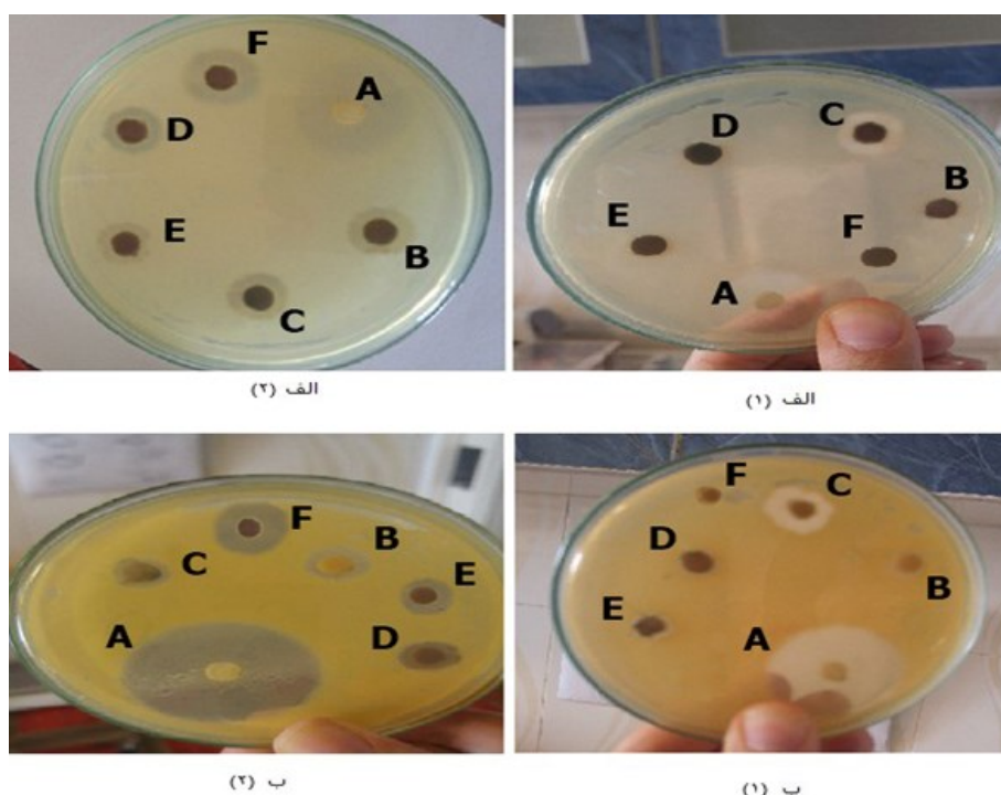
شکل ۶- هاله عدم رشد در محیط کشت با کاربرد عصاره نانوذره نعنای فلفلی، الف - ۱: استافیلوکوکوس اورئوس ، ۲: اشریشیا کلی ، ب ۱: باسیلوس سرئوس ، ۲: سالمونلا تیفی (A: کوآموکسیکلاو، B: غلظت ۱۰ میکروگرم بر میلی لیتر نانوذره شیریشا کلی، C: محلول نمک طلا، D: غلظت ۳۰ میکروگرم بر میلی لیتر نانوذره، E: غلظت ۶۰ میکروگرم بر میلی لیتر نانوذره و F: غلظت ۹۰ میکروگرم بر میلی لیتر نانوذره).
