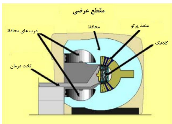
شکل ۳- نمایی از سیستم گامانایف به همراه بخش های مختلف آن (۶)
