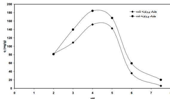
شکل ۵- تاثیر pH بر میزان جذب تعادلی اورانیوم توسط جلبک قهوه‌ای سیستوسریا ( غلظت اولیه ۳۵۰ ppm، غلظت جاذب g/L ۲، دما ۳۰°C، سرعت هم‌زدن ۱۵۰ rpm) (۱۳).
