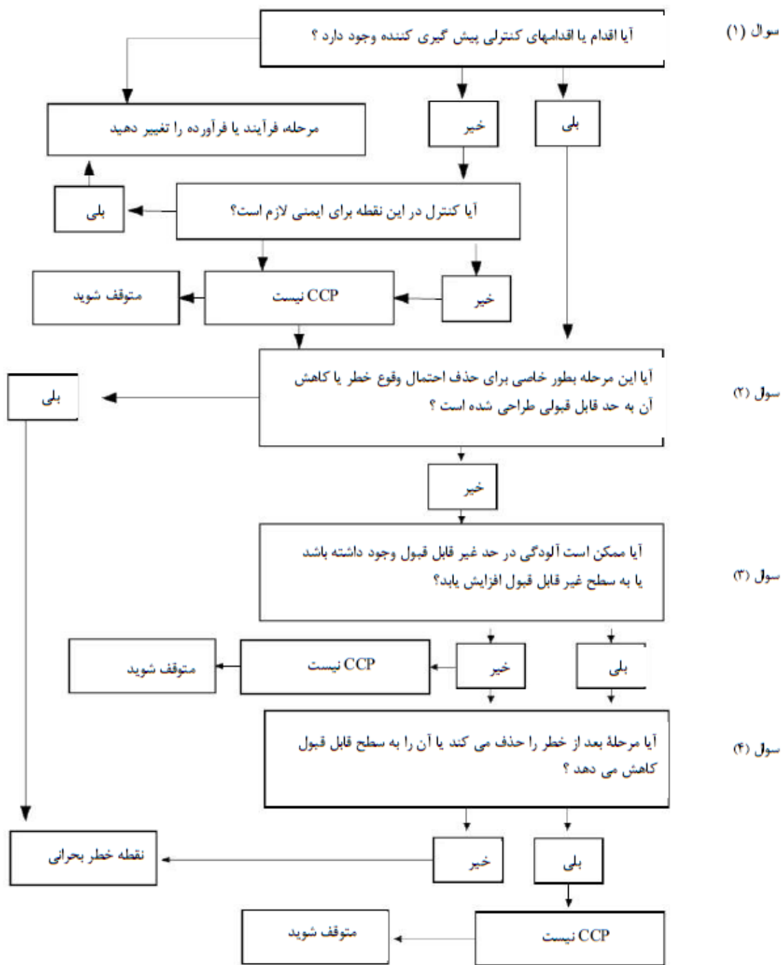
شکل ۱- نمونه‌ای از یک درخت تصمیم‌گیری برای مشخص کردن نقاط کنترل بحرانی
