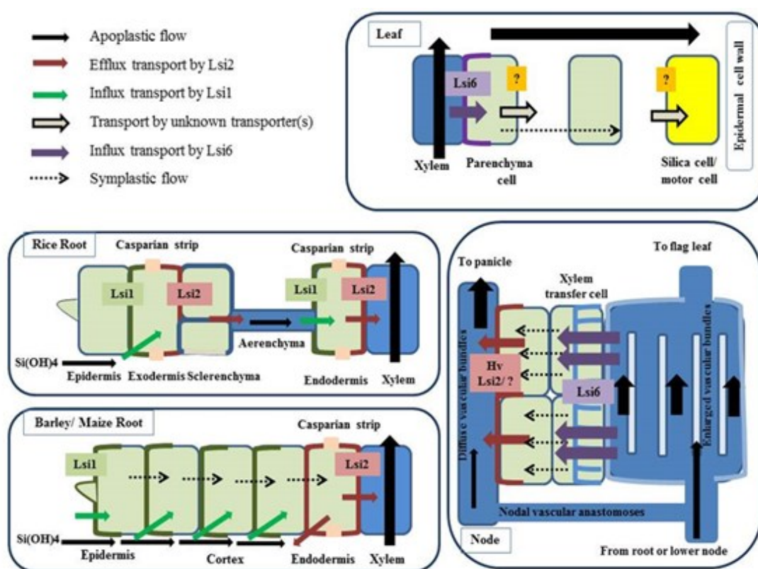
شکل ۲- نمایش سیستم انتقال سیلیسیم (Si) برای جذب، تخلیه در آوند چوبی و توزیع آن در گیاهان.
