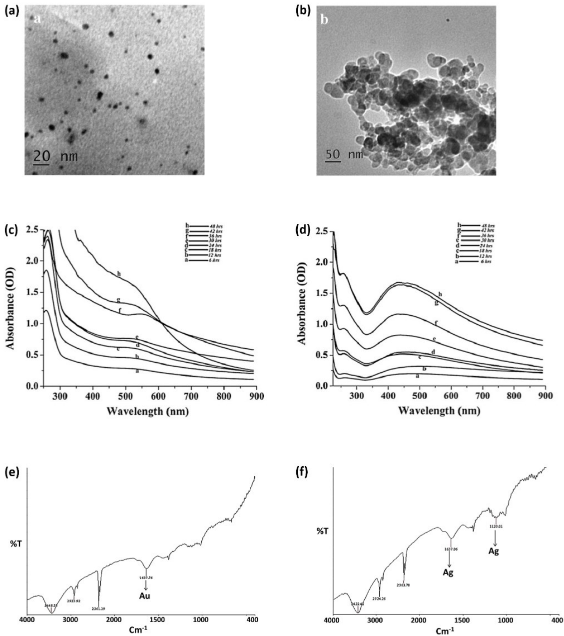
شکل ۴- تصاویر TEM نانوذرات طلا (a) و نقره (b) و طیف UV-Vis نانوذرات طلا (c) و نقره سنتز شده با قارچ C. albicans (Ahmad et al. 2013)، طیف FTIR نانوذرات طلا (e) و نقره سنتز شده با گیاه خرفه سا (Geethalakshmi and Sarada 2013)
