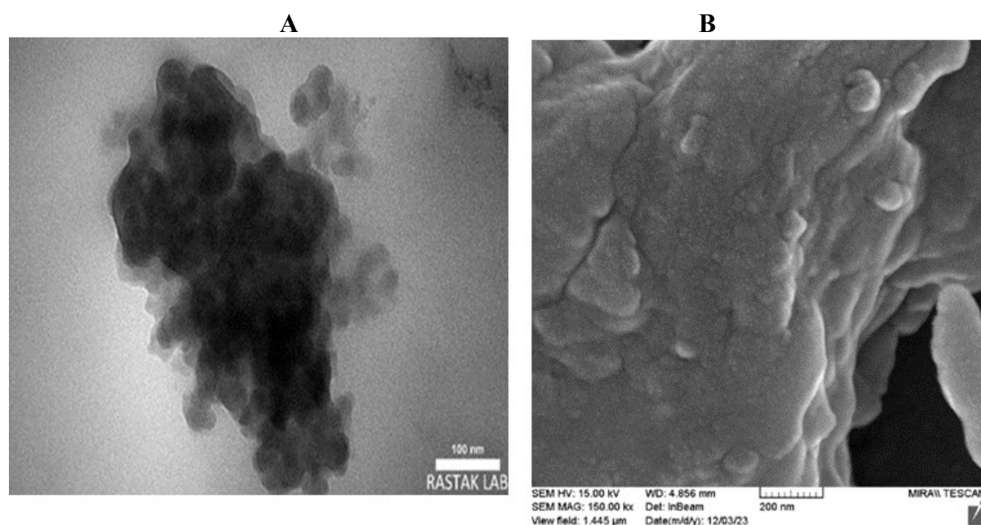
شکل ۳- (A) تصویر TEM از نانوحشره کش، (B) مورفولوژی SEM نانوحشره کش
