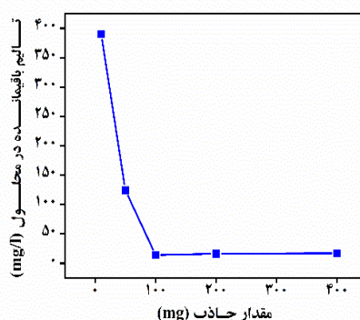
شکل ۳. نمودار تغییرات تالیم باقیمانده در محلول نسبت به مقدار جاذب
