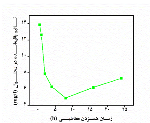
شکل ۴. نمودار تغییرات تالیم باقیمانده در محلول نسبت به زمان هم زدن مغناطیسی
